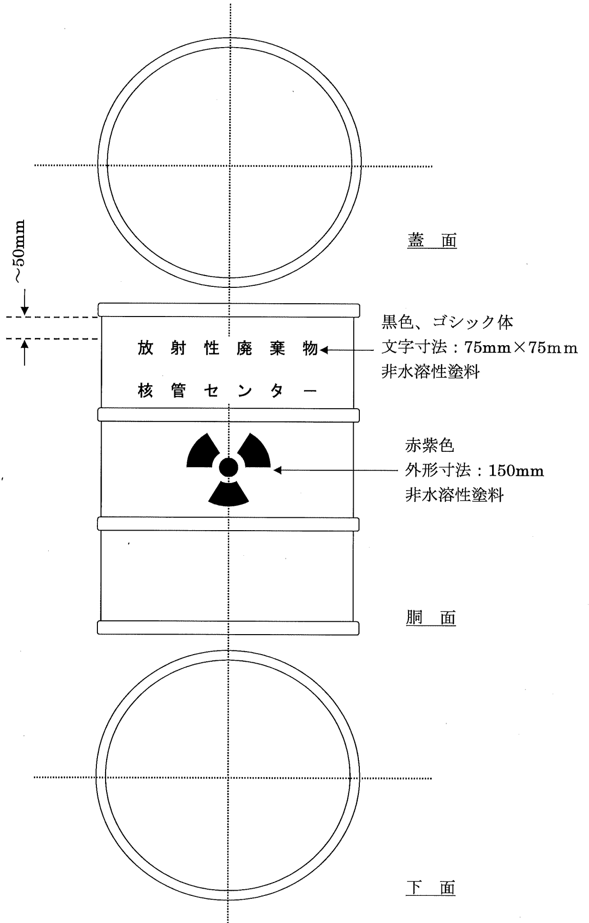
別添図1 文字、RIマークの印字
